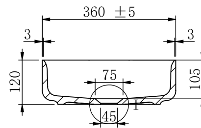
B-B
