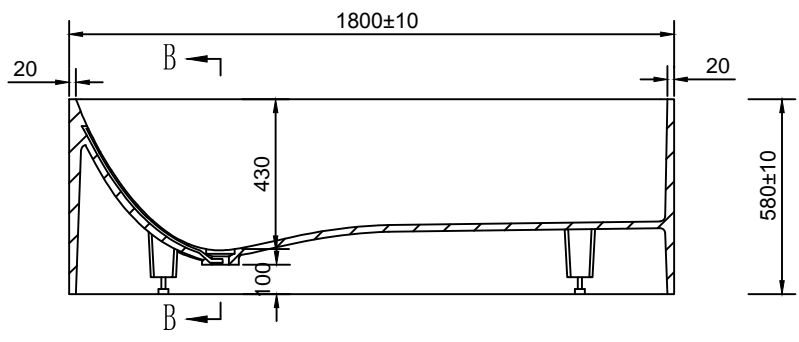
A-A
